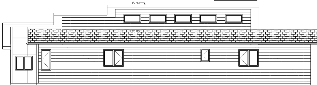
RIGHT ELEVATION
