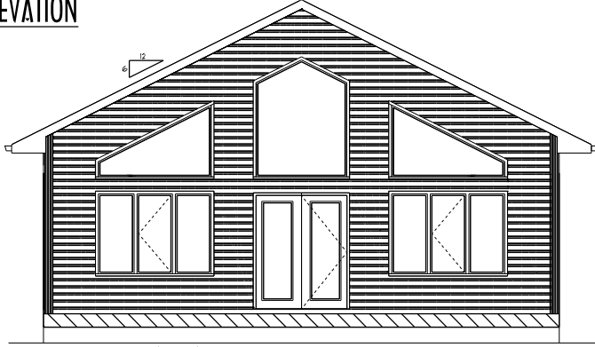
RIGHT ELEVATION
